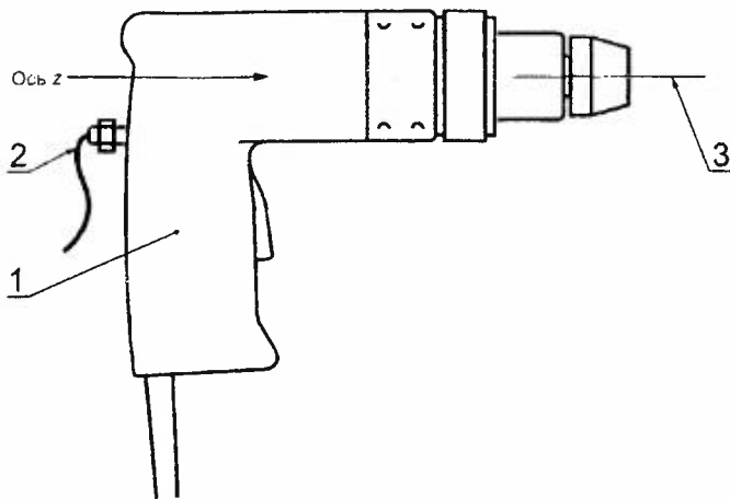
Рисунок 1 — Направление измерений, пример расположения и крепления вибропреобразователя
