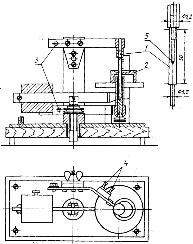
Рисунок 9 — Прибор для испытания горячим коническим сердечником
