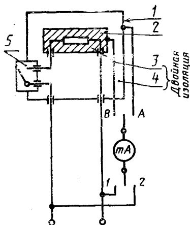
Рисунок 2 — Испытательный шуп
