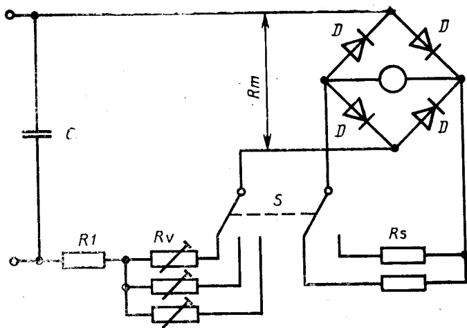
Рисунок 1А1 — Схема цепи для измерения тока утечки
