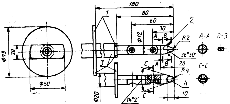
1—стопорная пластина; 2—цилиндрическая часть; 3—изоляционный материал
