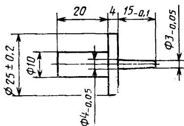
Рисунок 2 — Испытательный шуп
