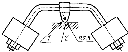
Рисунок 8 — Прибор для вдавливания шарика
