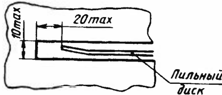
Рисунок 103 — Размеры прорези в столе
