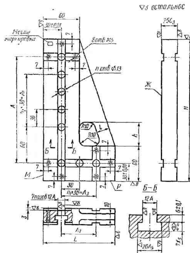
Поверхности М, Ж, Р — базы для контроля.
