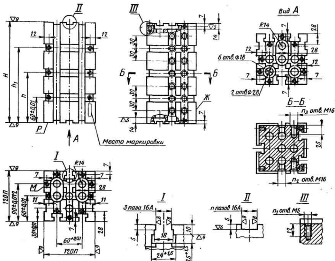
Поверхности М, Ж, Р — базы для контроля
